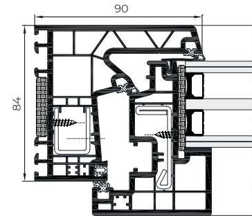
A 84 Hidden Sash Passivhausvhaus
