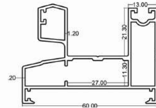
چهار چوب تک تیغه SINGLE BLADE FRAME
