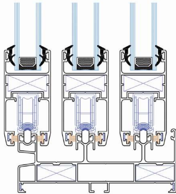
لیست برش سیستم ریلی نرمال اختصاصی تابریل ۶۰
