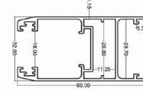
لنگه ریلی ۷۰ VENT PROFILE 70
