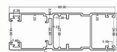
لنگه ریلی ۹۰ VENT PROFILE 90
