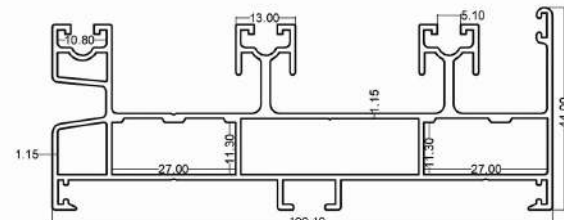
چهارچوب عرق گیر سه ریل 3 RAILS TAKEOUT FRAME
