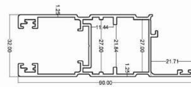
لنگه ریلی ۹۰ زهوار خور VENT ON RICETY A PLACE 90
